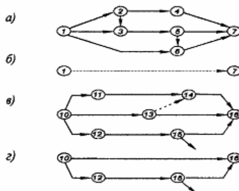
Рис. 3.14- Примеры укрупнения сетей: а, в — до укрупнения, б, г — после укрупнения
