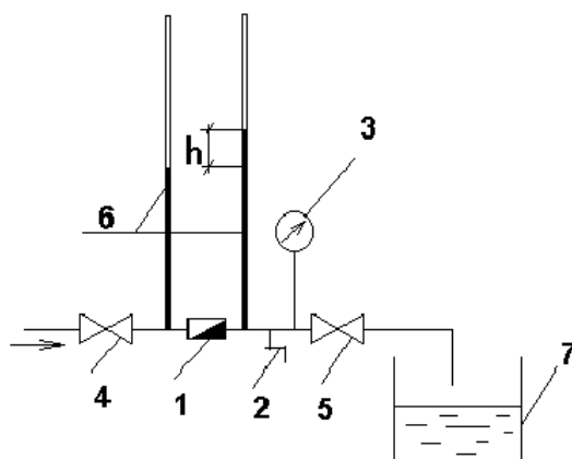
Рис.4.1. Схема установки
