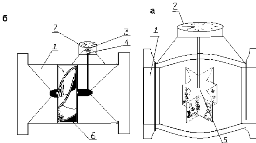
Рис 3.2. Скоростные счетчики воды а) крыльчатый; б) турбинный; 1-корпус; 2-циферблат; 3-счетный механизм; 4-магнитная муфта; 5- крыльчатка; 6-турбина.
