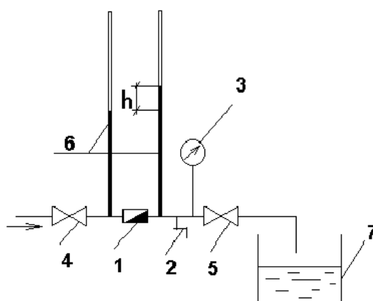
Рис.4.1. Схема установки
