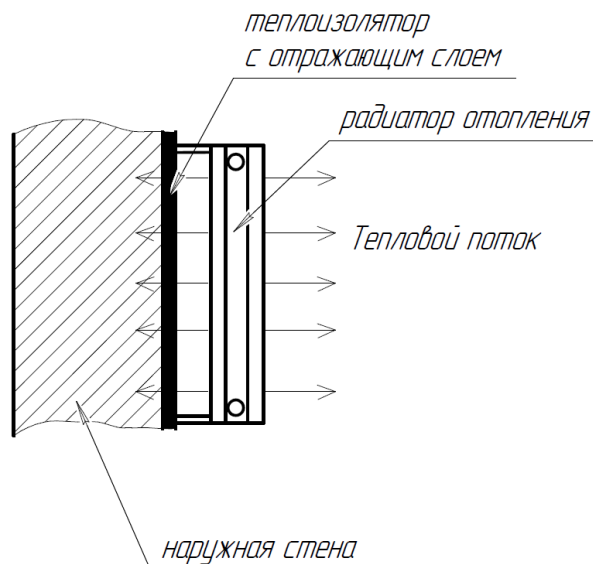
Рисунок 1. Общий вид смонтированного теплоотражателя
