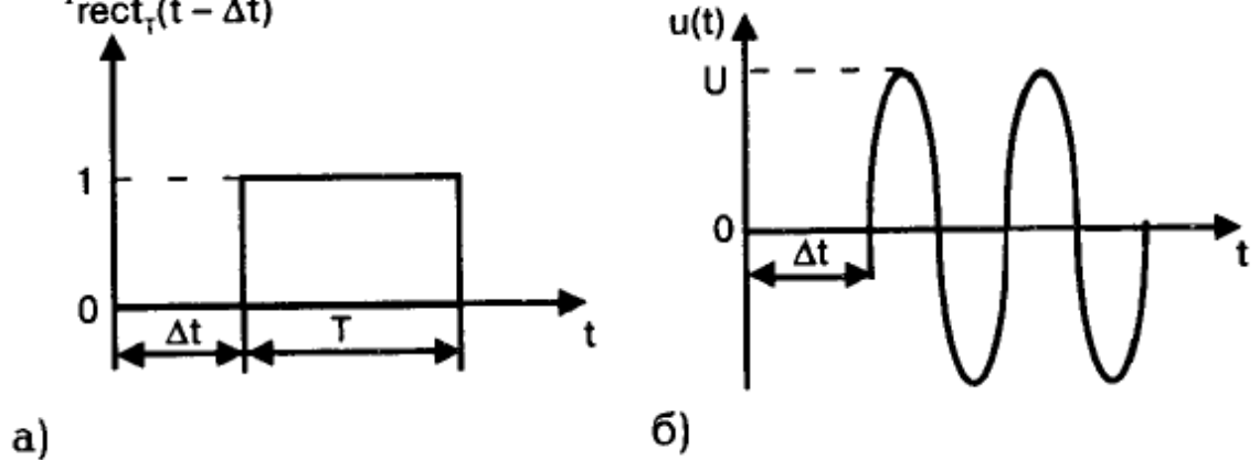
Рис. 7.2 Виды сигналов: а) электрический сигнал; б) синусоидальное колебание
