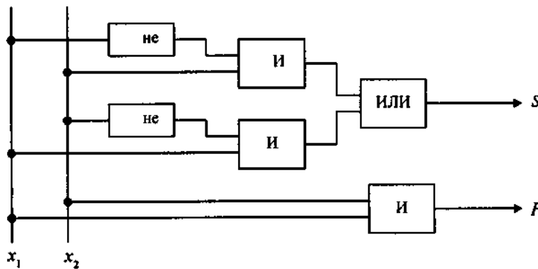
Рис 4.5. Логическая схема сумматора
