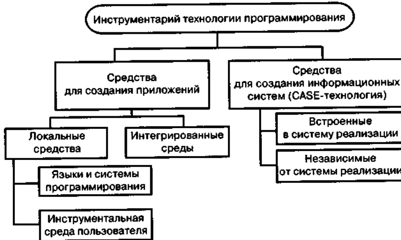
Рис.54. Классификация инструментальных средств программирования
