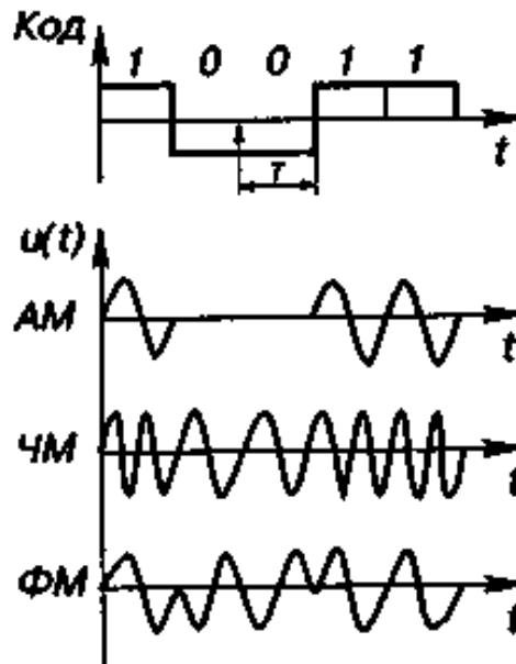
Рис 7.3. Виды двоичных сигналов
