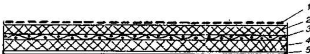
Рисунок 5 – Схема поперечного сечения полимербитумного рулонного материала:
