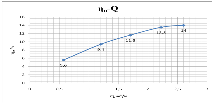
Рис.3.4.- Энергетическая характеристика
