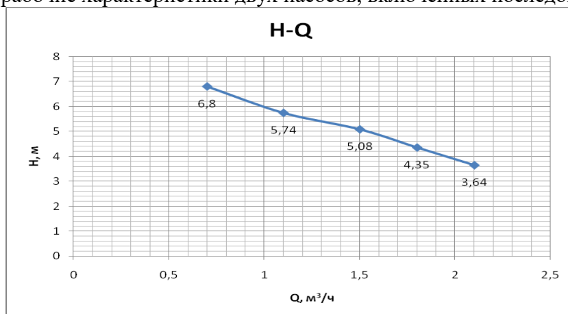
Рис.2.2.- Напорная характеристика
