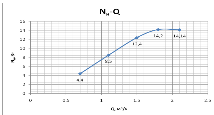
Рис.2.3.- Мощностная характеристика
