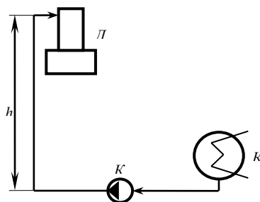
Рис.3.2. Схема установки
