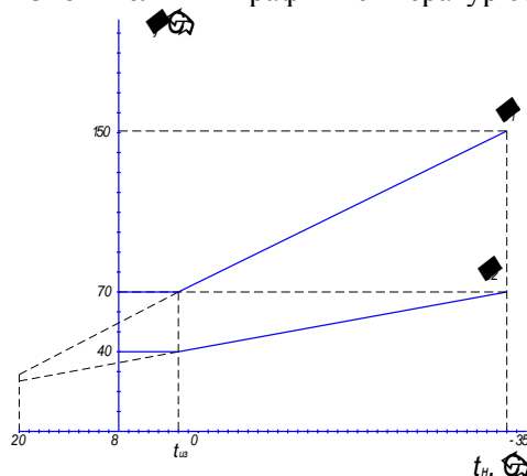
Рисунок 2 – Отопительно-бытовой график температур сетевой воды
