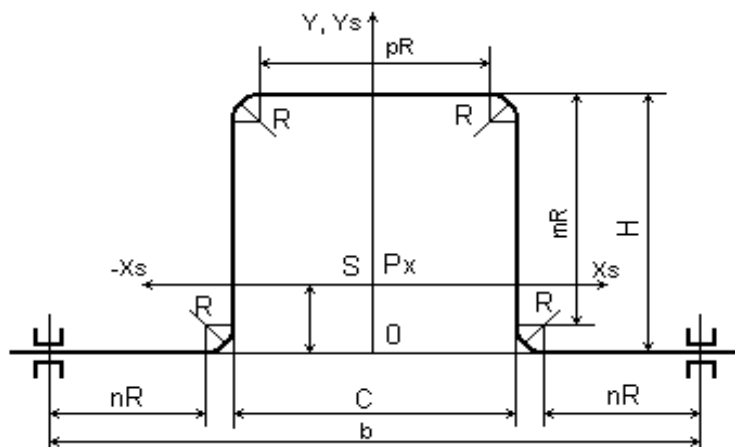
Рисунок 1 – Расчетная схема П образного компенсатора.
