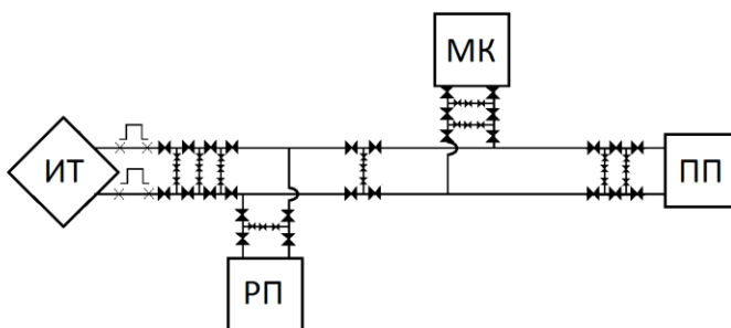
Рисунок 1 – Монтажная схема
