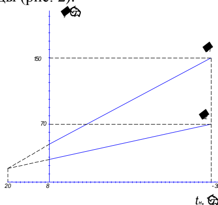
Рисунок 1 – Отопительный график температур сетевой воды
