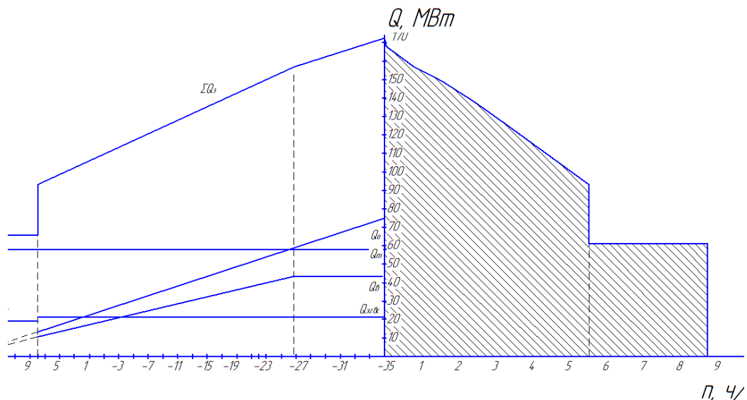
Рисунок 1 – График продолжительности тепловых нагрузок.
