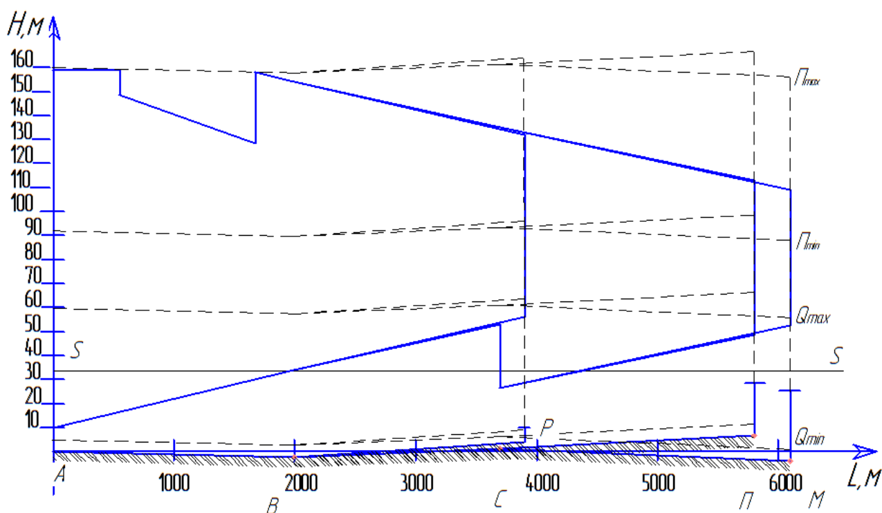
Рисунок 2 – Пьезометрический график
