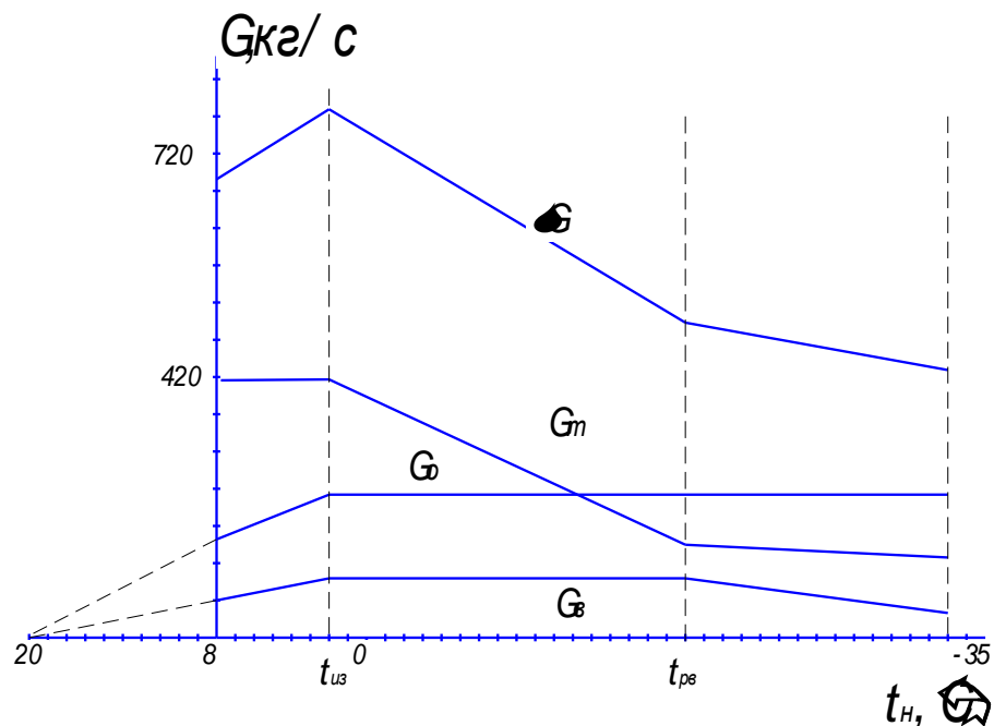
Рисунок 6 – График суммарных расходов сетевой воды.
