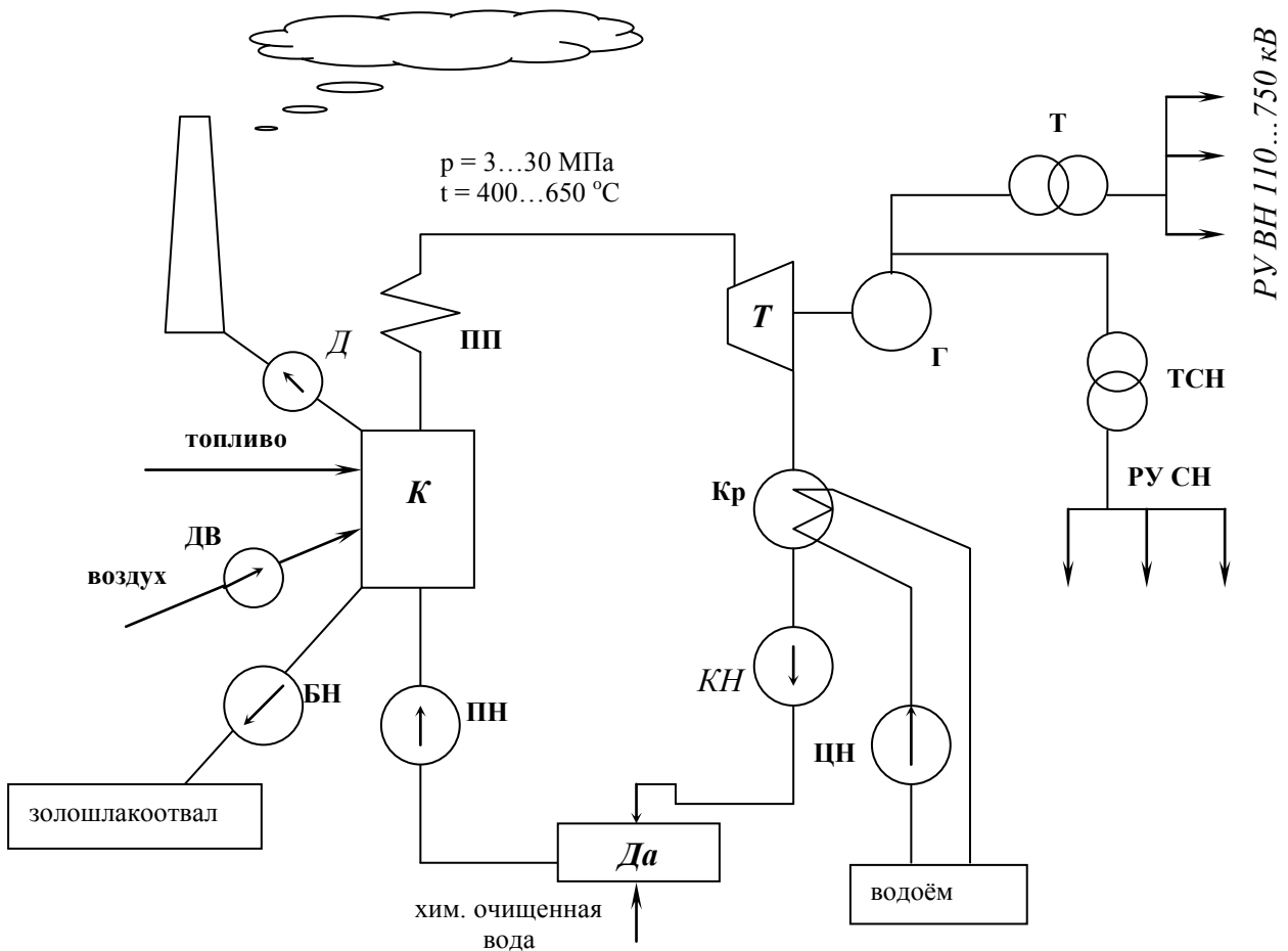
Рис.4.1. Технологическая схема КЭС
