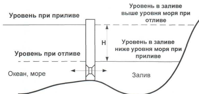
Рис.7.4. Схема создания напора ПЭС
