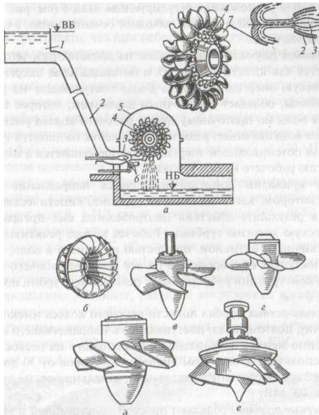
Рис.7.1. Общие виды рабочих колес гидротурбин: а - принцип работы и общий вид ковшовой турбины: 1 - бассейн верхнего уровня (бьефа); 2 - турбинный трубопровод; 3 - сопло; 4 - рабочее колесо; 5 - кожух; б - регулировочная игла; 7 - лопасти (ковши);
