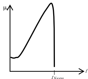
Рис. 1.34. Зависимость \mu_r = f(t^\circ) для магнитных материалов
