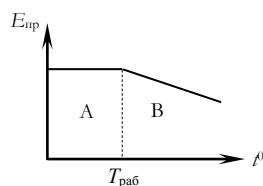
Рис. 1.30. Зависимость E_{пр} = f(t^\circ) для твёрдых диэлектриков: А – область электрического пробоа; В – область теплового пробоа
