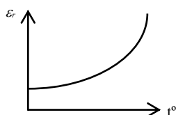
Рис. 1.15. Зависимость \epsilon_r = f(t^\circ) для твёрдых тел с ионной структурой и неплотной упаковкой частиц
