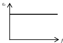
Рис. 1.9. Зависимость \varepsilon_r = f(f) для неполярного жидкого диэлектрика
