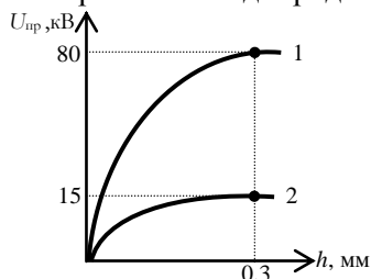
Рис. 1.28. Зависимость U_{пр} от однородности электрического поля для неорганического стекла
