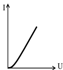
Рис. 1.19. Вольтамперная характеристика жидкого диэлектрика
