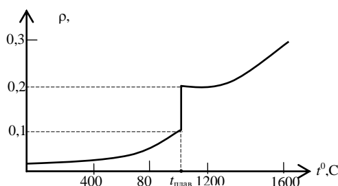
Рис. 1.29. Зависимость \rho от t °С для меди
