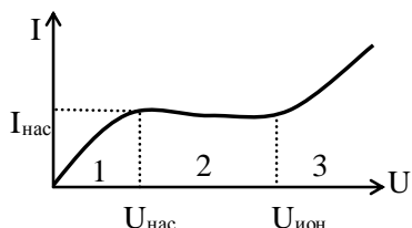
Рис. 1.18. Вольтамперная характеристика газообразного промежутка
