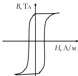
Рис. 1.37. Прямоугольная петля гистерезиса
