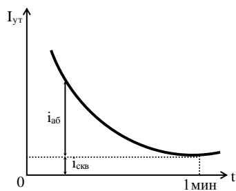
Рис. 1.17. Изменение I_{\text{ут}} во времени
