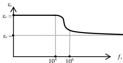
Рис. 1.11. Зависимость \varepsilon_r от частоты электрического поля для полярных жидкостей
