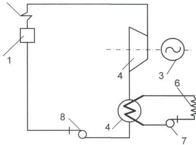
Рис. 2. Тепловая схема простейшей ТЭЦ
