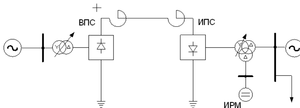
Рисунок №1 Условная схема системы и распределения электроэнергии
