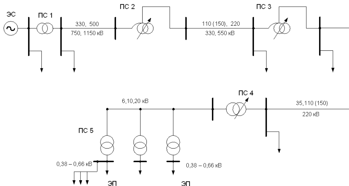
Рисунок №1 Условная схема системы и распределения электроэнергии
