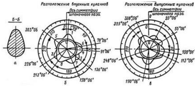
Рис. 2.3. Приспособление для контроля профиля кулачков и опорных шеек распределительного вала: а - профиль кулачка, б - расположение впускных кулачков; в - расположение выпускных кулачков; Вп - впускной кулачок; Вып - выпускной кулачок; 1 - основание приспособления; 2,9 - центры; 3 - диск с градуировкой, град; 4 - указательная стрелка, закрепленная на шейке распределительного вала; 5 - ножка индикатора; 6 - стойка индикатора; 7 - индикатор, 8 - распределительный вал.
