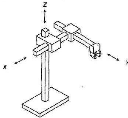
Рис. 2. Манипулятор с декартовой системой координат и его рабочая зона
