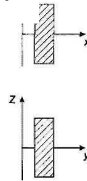
Рис. 2. Манипулятор с декартовой системой координат и его рабочая зона
