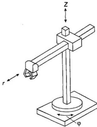
Рис. 3. Манипулятор с цилиндрической системой координат (а) и его рабочая зона (б)
