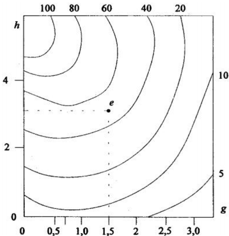
Рис. 12. Графики изолюксы
