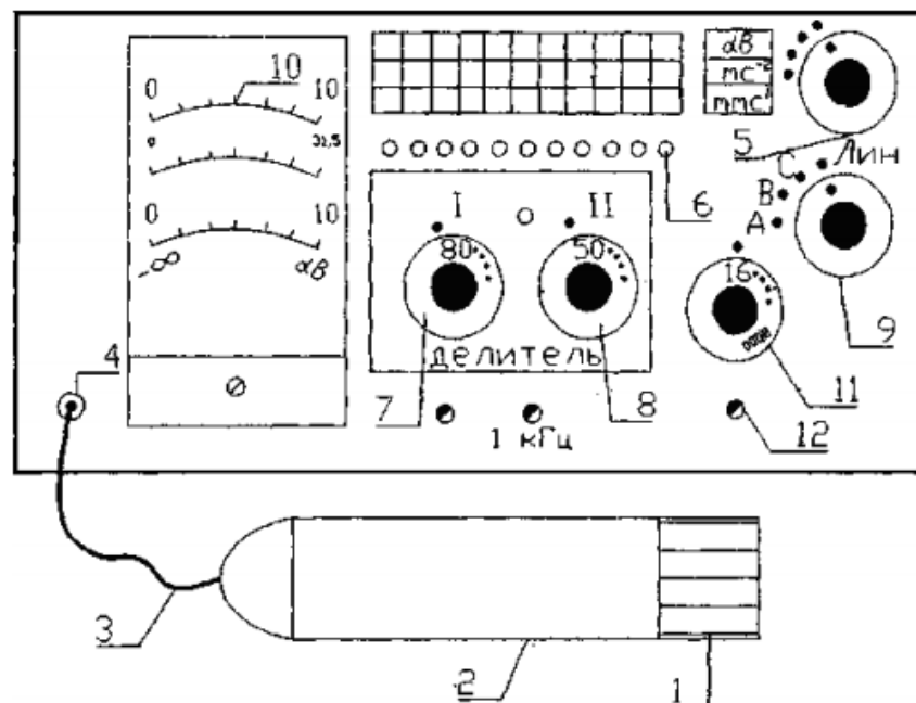
Рис. 3. Расположение ручек
