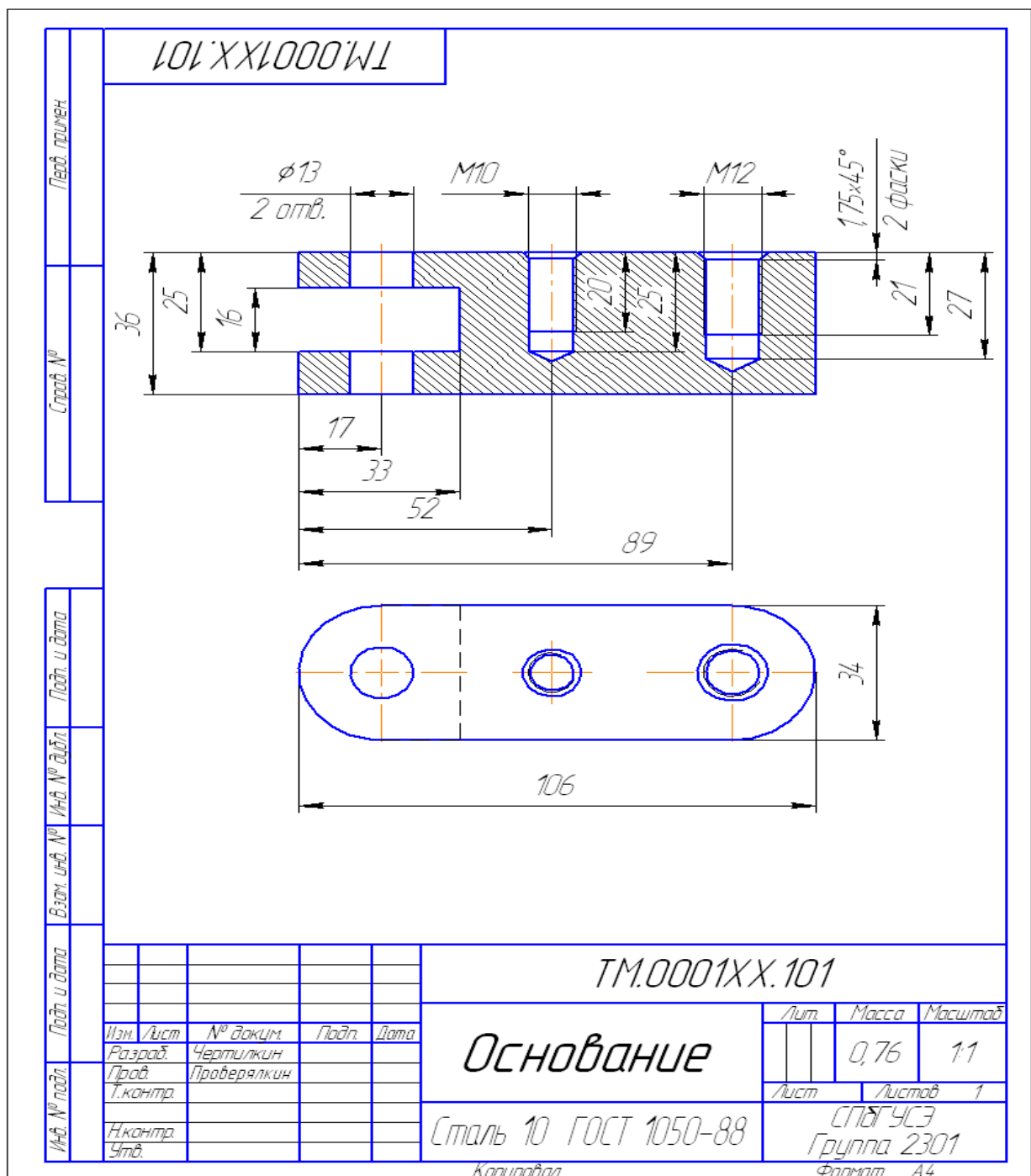
Рисунок 5. – Чертеж детали.
