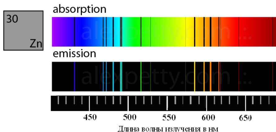
Спектры поглощения и излучения атомов цинка
