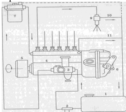
Рис. 1- Топливная система с механическим управлением подачи топлива:
