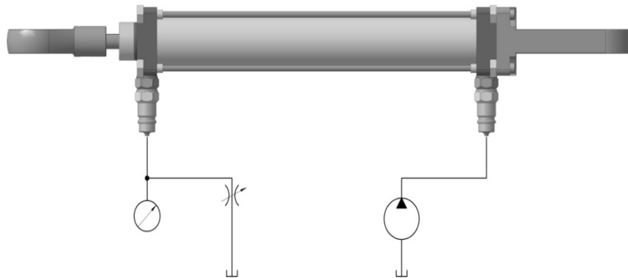
Рис. 6.1. – Практический пример: Гидроцилиндр со стяжными шпильками.
