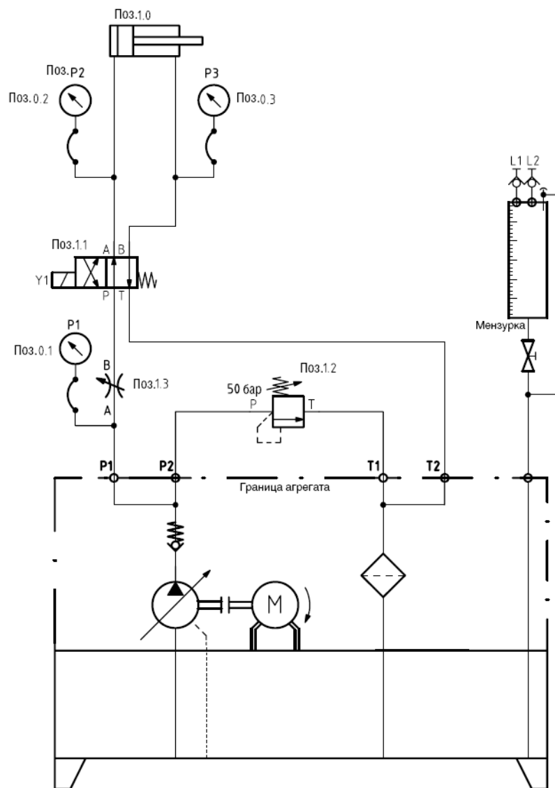
Рис.7.2. – Гидравлическая схема: Гидроцилиндр с регулируемой скоростью хода.
