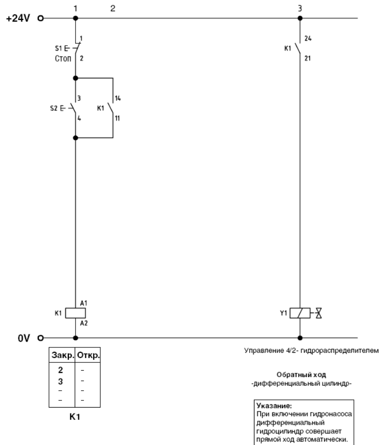
Рис.7.3. – Электросхема к гидравлической схеме на рисунке 7.2.
