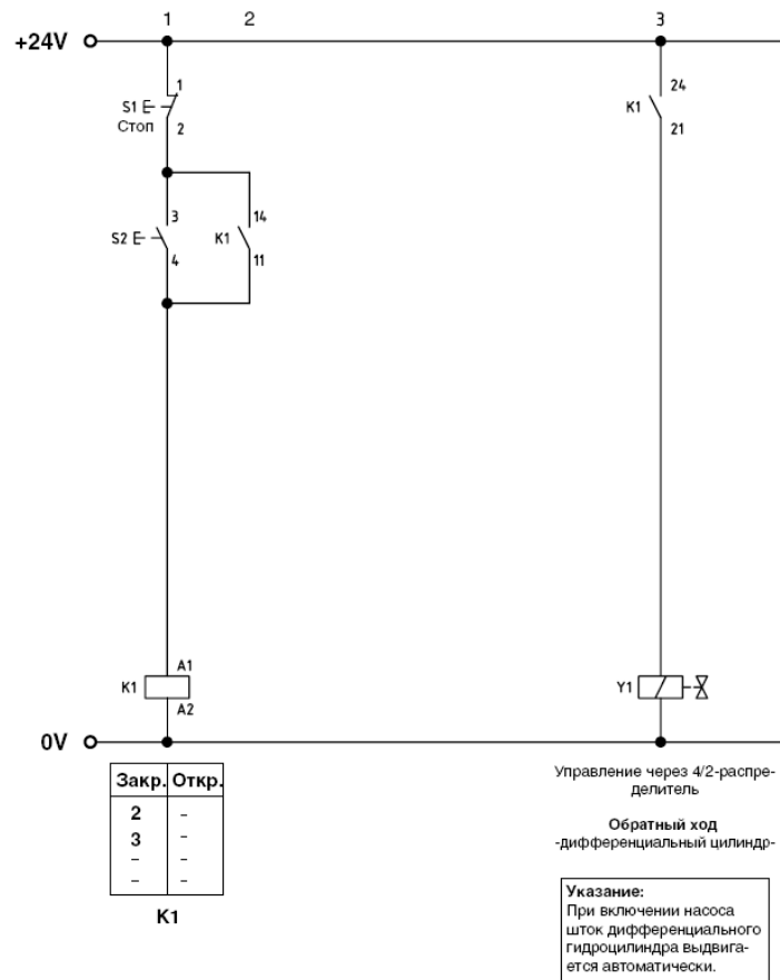
Рис.6.3. – Электросхема к гидравлической схеме.
