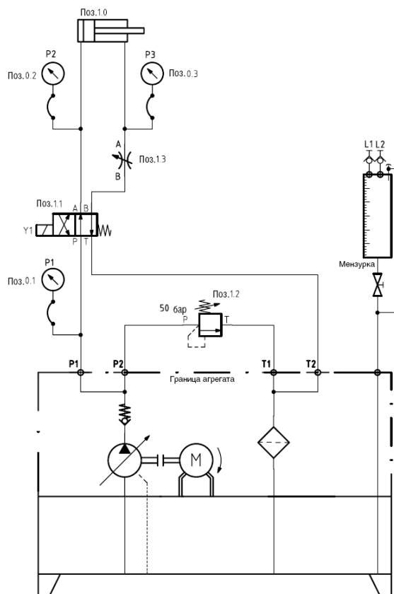
Рис.6.2. – Гидравлическая схема: Гидроцилиндр с регулируемой скоростью хода.
