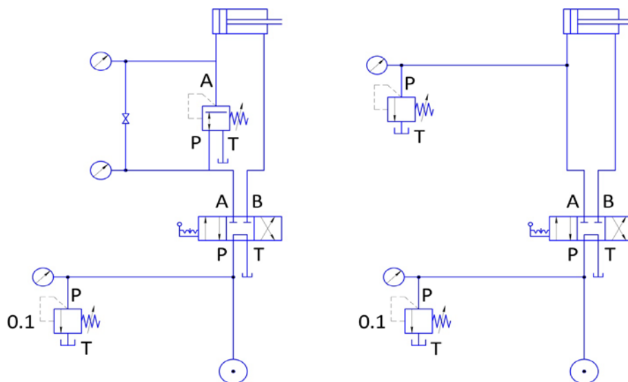
Рис.4.4. - Гидравлическая принципиальная схема. Переплетный пресс.
