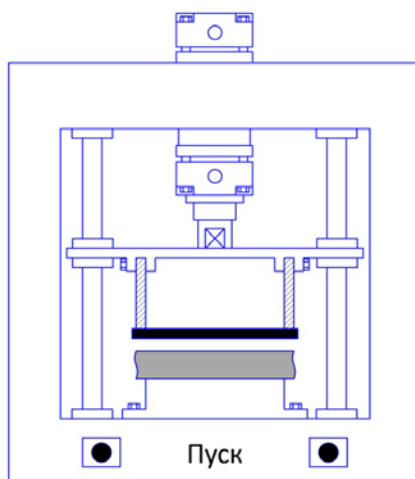
Рис.4.3. – Переплетный пресс
