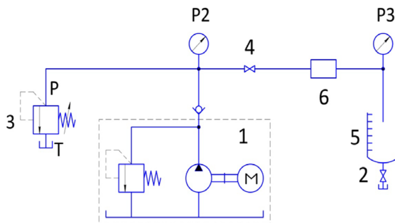
Рис.2.2. - Гидравлическая принципиальная схема проливки трубопроводов и гидроаппаратов
