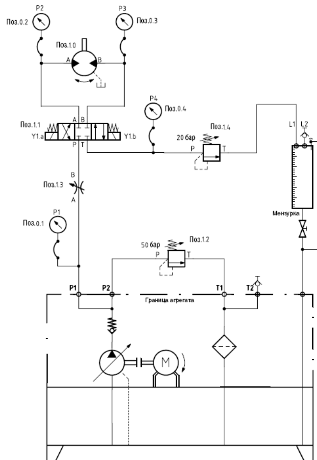
Рисунок 8.2. – Гидравлическая схема.
