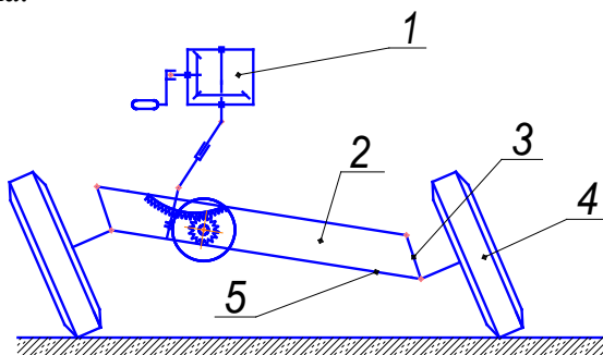
Рис .5. Схема заднего моста грейдера ДЗ -1: 1 – механизм наклона колес, 2 – штанга, 3 – кривошип, 4 – колесо, 5 - балка
