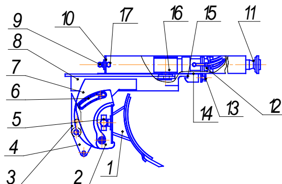
Рис. 10. Рабочий орган грейдера СД-107:
