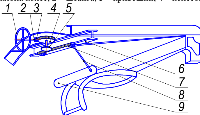
Рис.6. Механизм выноса отвала в сторону грейдера ДЗ-1: 1-штурвал; 2-вал; 3-червяк; 4-червячное колесо; 5-шестерня; 6-направляющая балка; 7-зубчатая рейка; 8-тяги; 9-тяговая рама.
