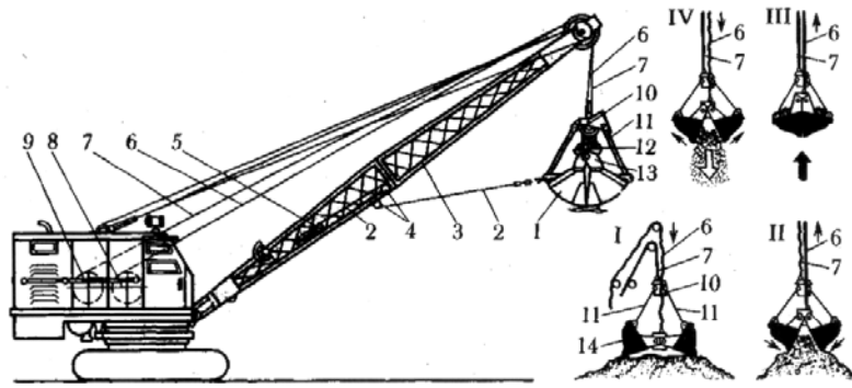
Рис. 10. Схема рабочего оборудования грейфера: 1 - ковш; 2, 6, 7 - канаты; 3 - стрела; 4, 12 - блоки; 5 - груз; 8, 9 - барабаны; 10, 13 - головки; 11 - тяги; 14 - челюсти; I...IV — положения грейфера
