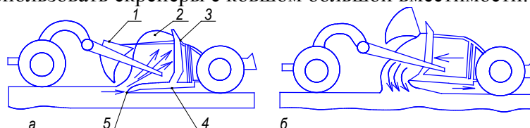
Рис.4. Схема скрепера, заполняемого тяговым усилием
