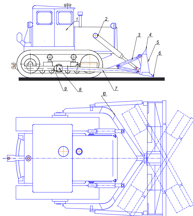
Рис. 4. Бульдозер ДЗ-18
