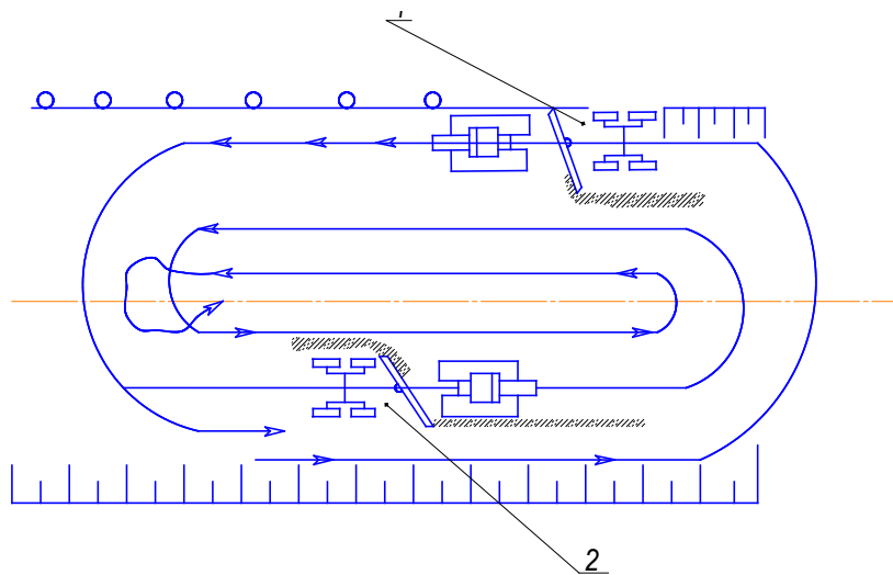
Рис.17 Схема одновременной работы двух грейдеров; 1, 2 - грейдеры
