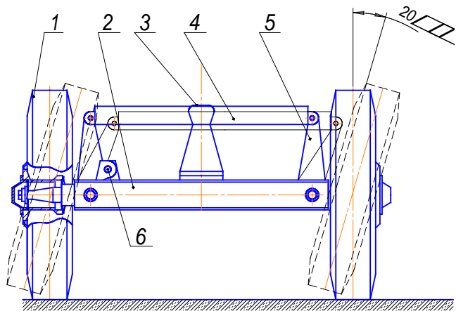
Рис.3. Передний мост грейдера ДЗ-1: 1 – колесо, 2 - балка, 3 – шаровая пята, 4 – поперечина, 5 – кривошип, 6 - чека
