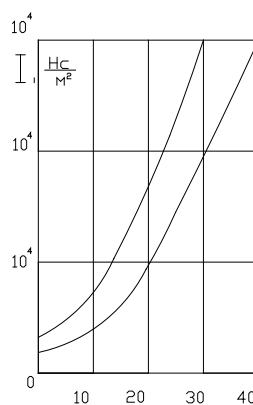
Рис. 3 - Содержание глинистых частиц в %.
