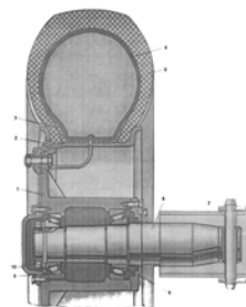
Рис. 12. Колесо скрепера
