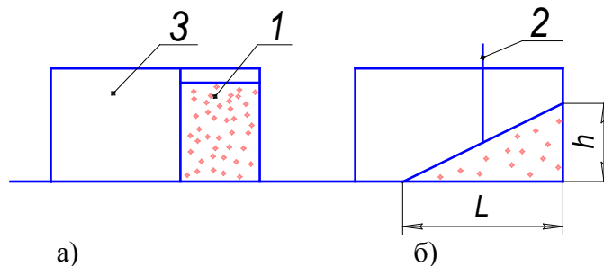
Рисунок 3 - Прибор Литвинова для определения угла естественного откоса песка. 1 – малый отсек, 2 – задвижка, 3 – большой отсек.
