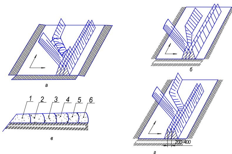
Рис. 16. Схемы укладки валиков грунта в теле насыпи:
