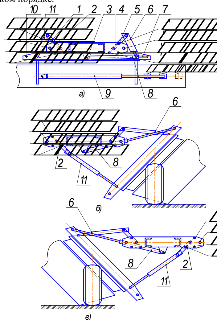
Рис. 12.Механизм подъема, опускания и бокового выноса отвала грейдера СД-107:
