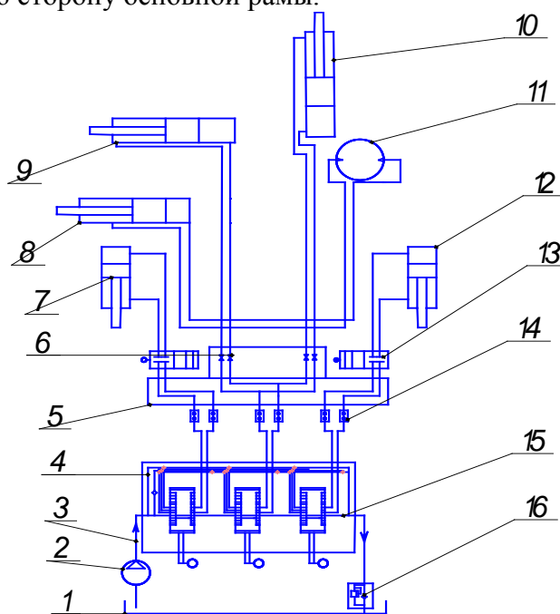
Рис. 13 Гидросистема грейдера СД-107:
