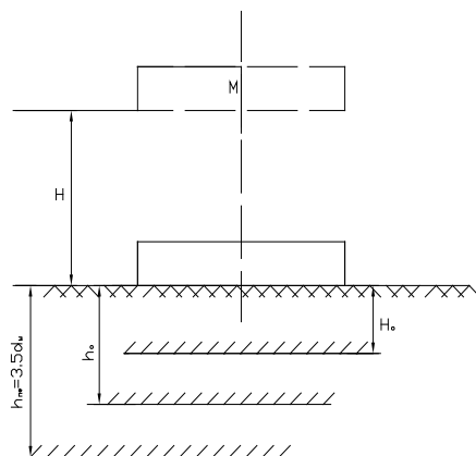
Рис. 1 - Расчетная схема процесса уплотнения грунта при трамбовании.
