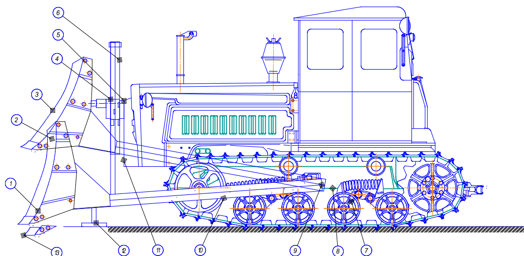
Рис.1. Бульдозер ДЗ-29.
