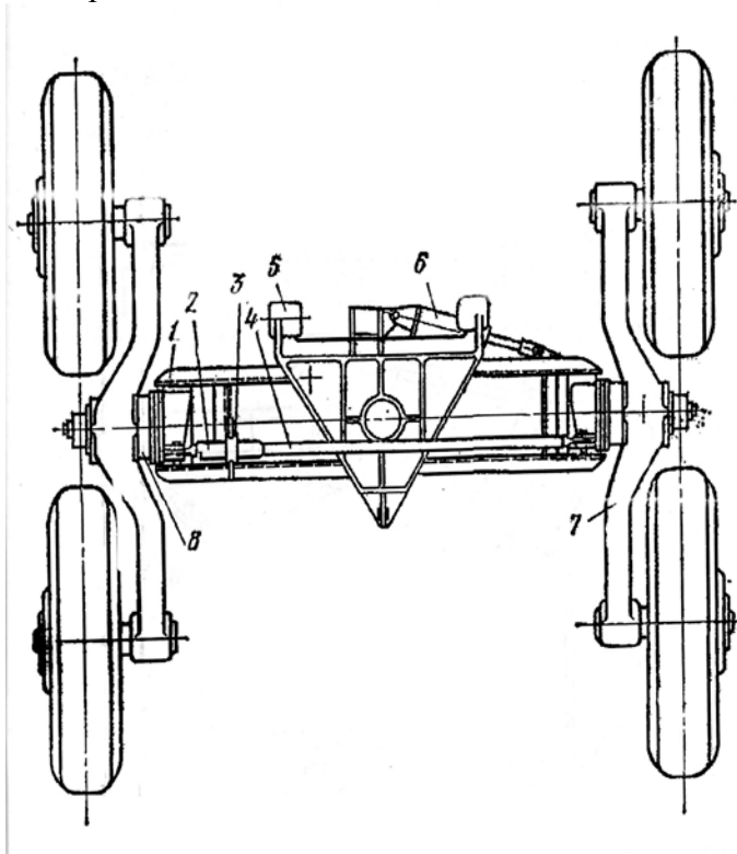
Рис.11. Задний мост грейдера СД-107:
