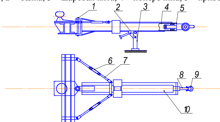
Рис.4. Дышло грейдера ДЗ-1: 1,8-шкворни; 2-фиксатор; 3-стойка; 4-штифт; 5-вкладыш; 6-натяжная муфта; 7-тяги; 9-прицепная серьга; 10-балка.
