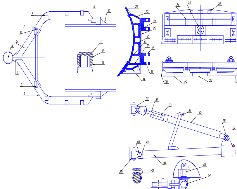
Рис. 6. Сборочные единицы бульдозера ДЗ-18
