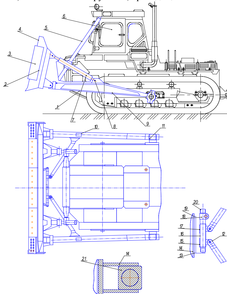
Рис.3. Бульдозер ДЗ-59
