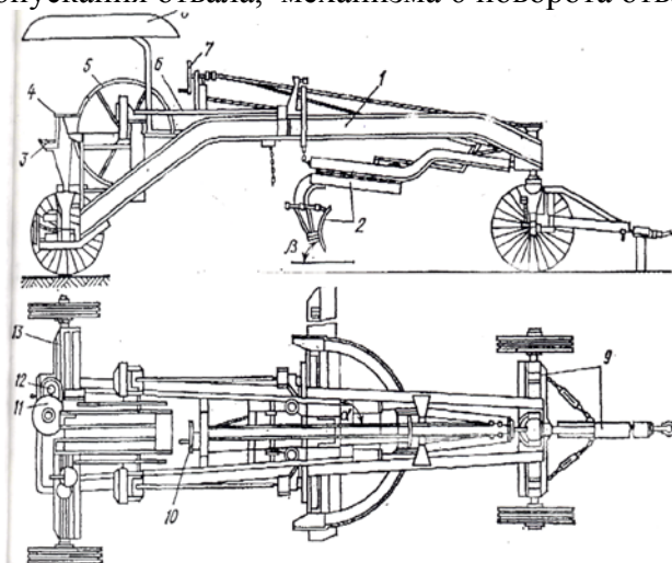
Рис. 1. Грейдер ДЗ-1:
