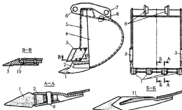
Рис. 14. Ковш обратной лопаты экскаватора ЭО-3322Д:
