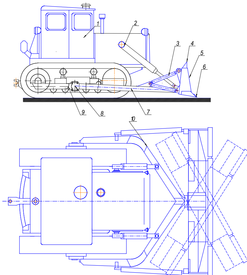
Рис. 5. Бульдозер ДЗ-18
