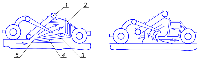
Рис. 5. Схема скрепера с элеваторной загрузкой.
