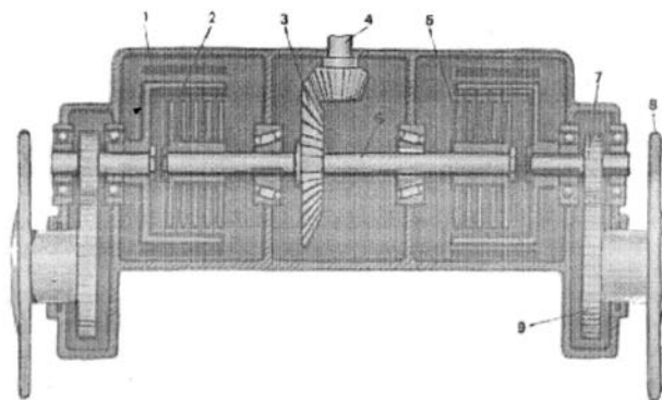
Рис.19. Схема заднего моста с фрикционным механизмом поворота:
