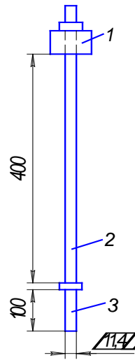
Рисунок 2 - Динамический плотномер :
