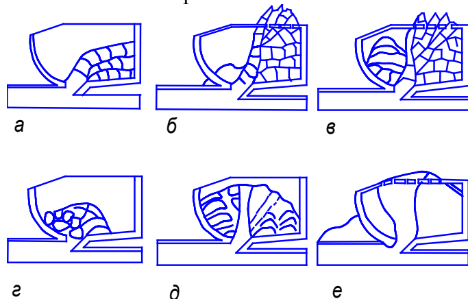
Рис. 8. Схема наполнения ковша грунтом а, б, в- связным; г, д, е- малосвязным
