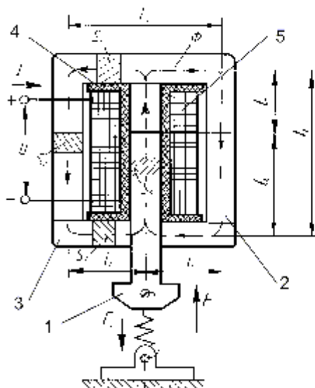
Рис. 2.21. Конструктивная схема электромагнита 1) втяжной якорь; 2) сердечник магнитопровода; 3) ядро (крышка) сердечника; 4) каркас катушки; 5) обмотка катушки
