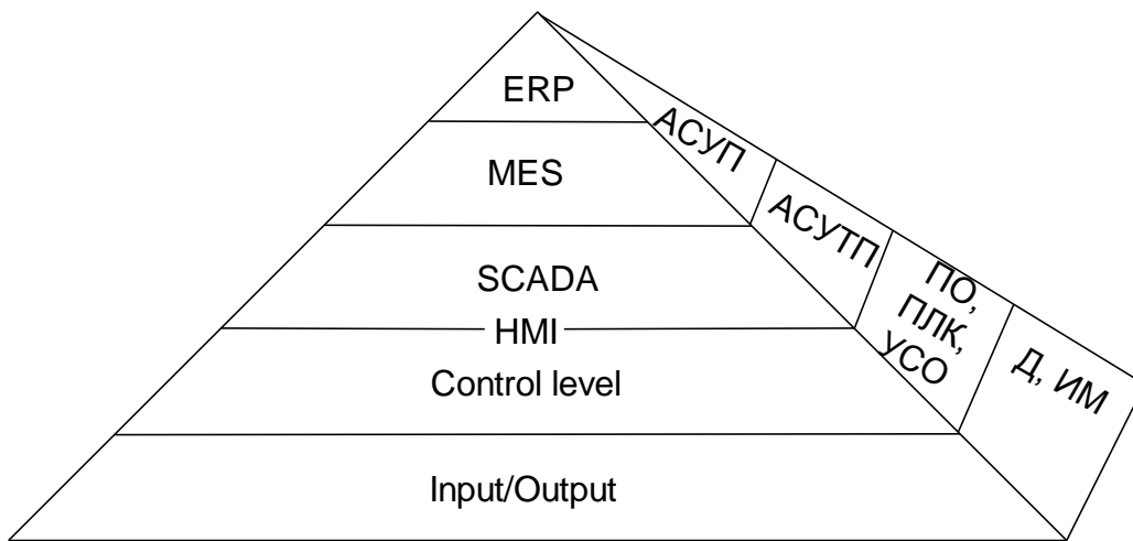
Рис. 2. Пирамида управления современным производством.
