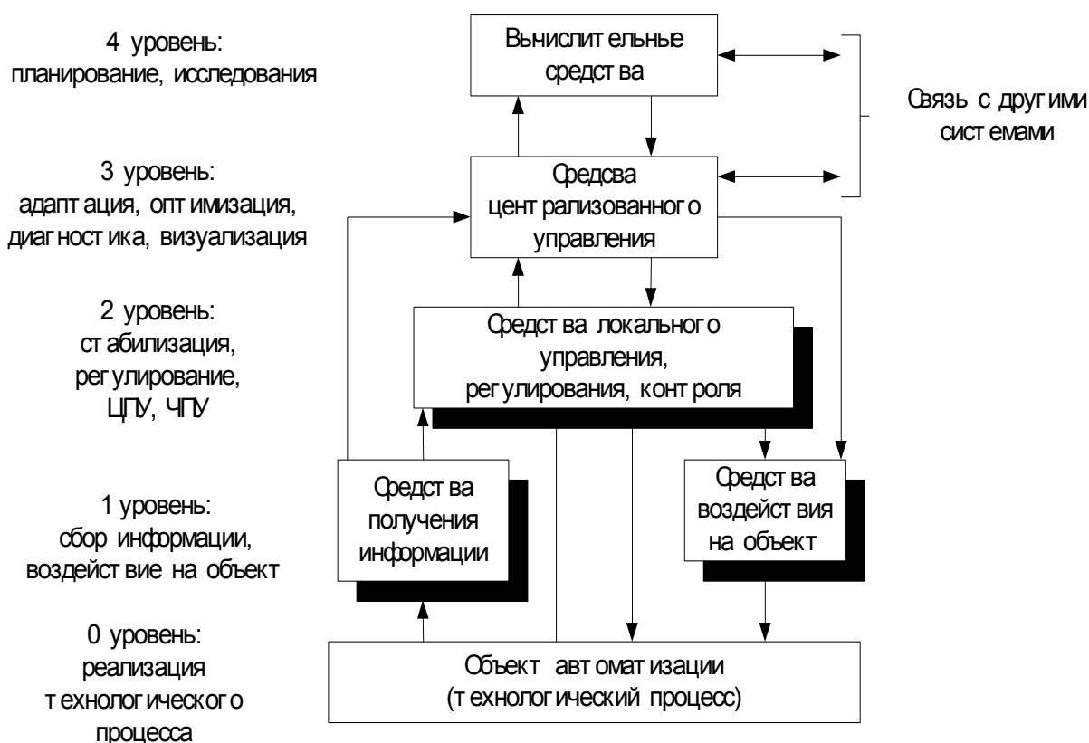
Рис. 1. Иерархия ГСП
