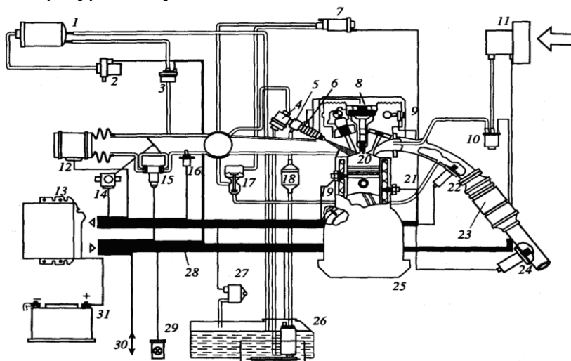
Рис.8.1. Компьютерная система управления работой бензинового двигателя
