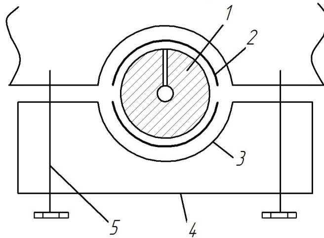
Рис.2.3. Постель блок-картера
