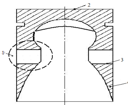
Рис.2.1. Поршень
