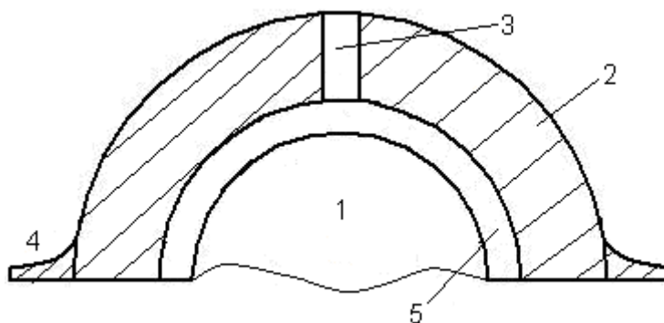
Рис.2.2. Конструкция вкладыша
