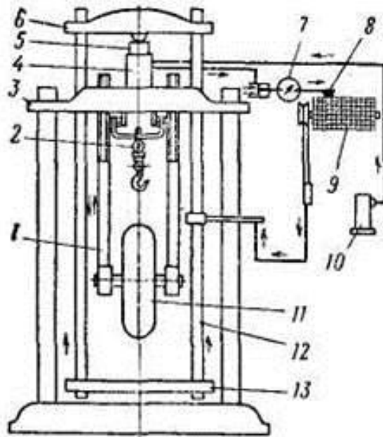
Рис. 6.1 Стенд ОПШ-30
