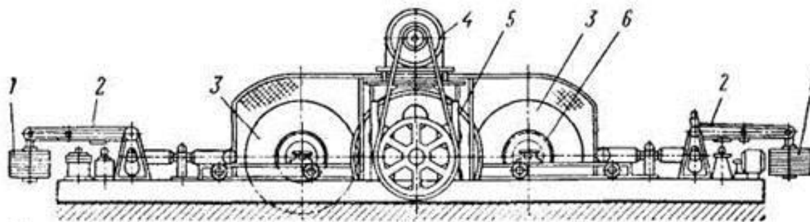
Рис. 6.5. Шинообкатный станок
