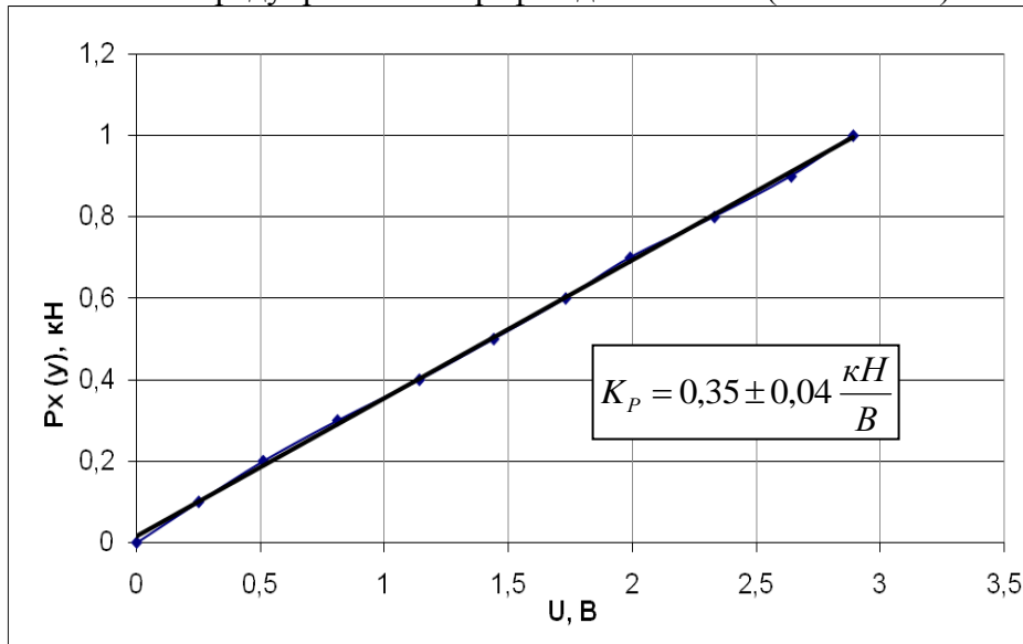
Градуировочный график датчика силы (тензовена)
