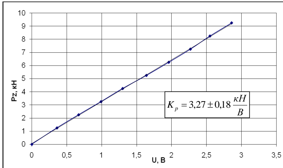
Градуировочный график датчика силы (тензовена)
