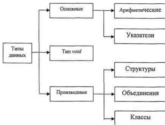
Рис. 2 Структура типа данных языка Си++
