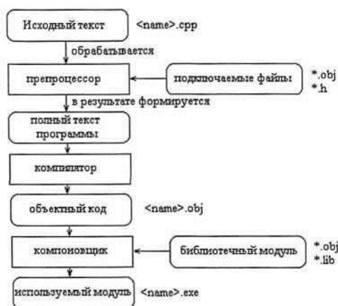
Рис.1 Структура процесса компиляции
