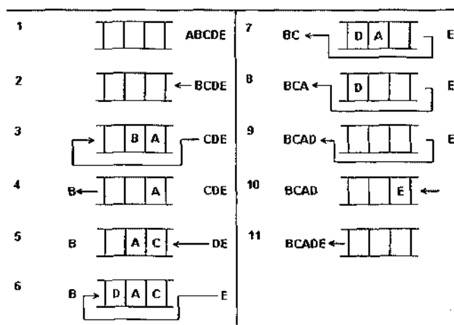
Рис. 4.2. Состояния дека в процессе изменения.
