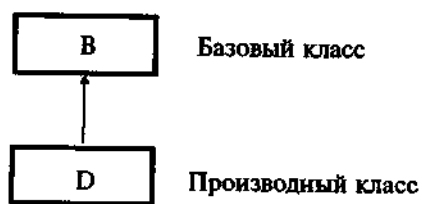
Рис. 4.1. Отношение наследования
