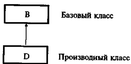
Рис. 4.1. Отношение наследования
