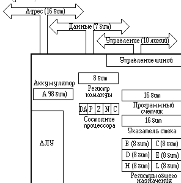
Рис. 1. Микропроцессор Intel 8080.
