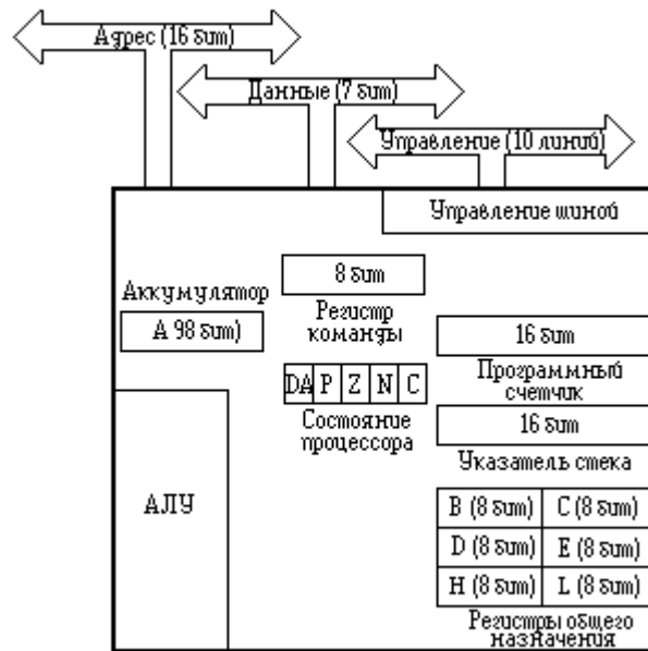
Рис. 1. Микропроцессор Intel 8080.
