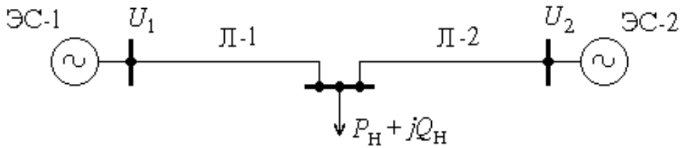
Рис. 1. Схема ЭЭС
