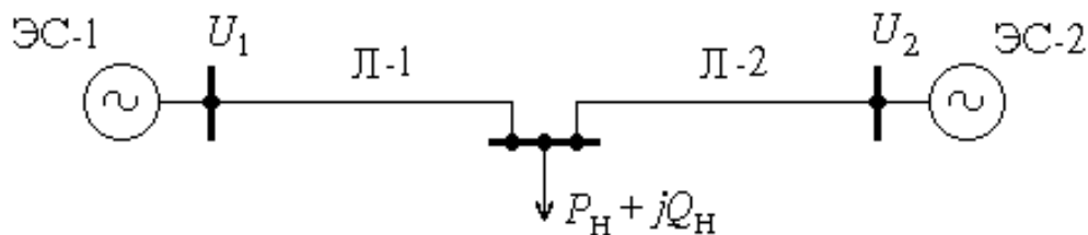
Рис. 1. Схема ЭЭС
