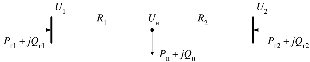
Рис.2. Схема замещения ЭЭС
