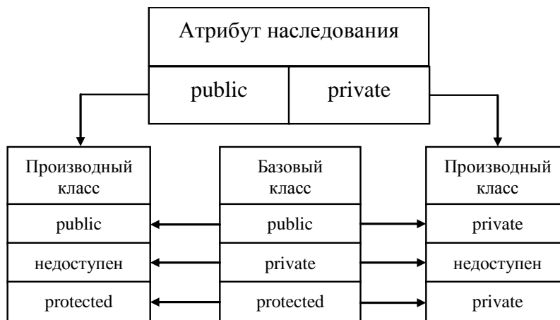
Рисунок 5.1 – Области видимости компонент класса
