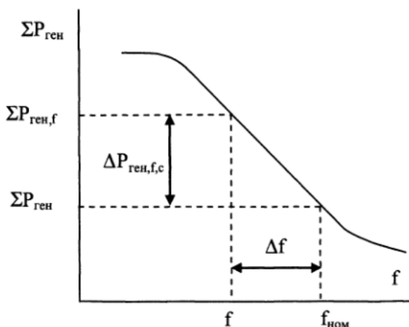
Рис. Частотная характеристика генерирующей энергосистемы
