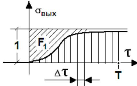
Рис. 10. Преобразование экспериментальной кривой разгона аperiodического звена второго порядка при использовании метода Симою.
