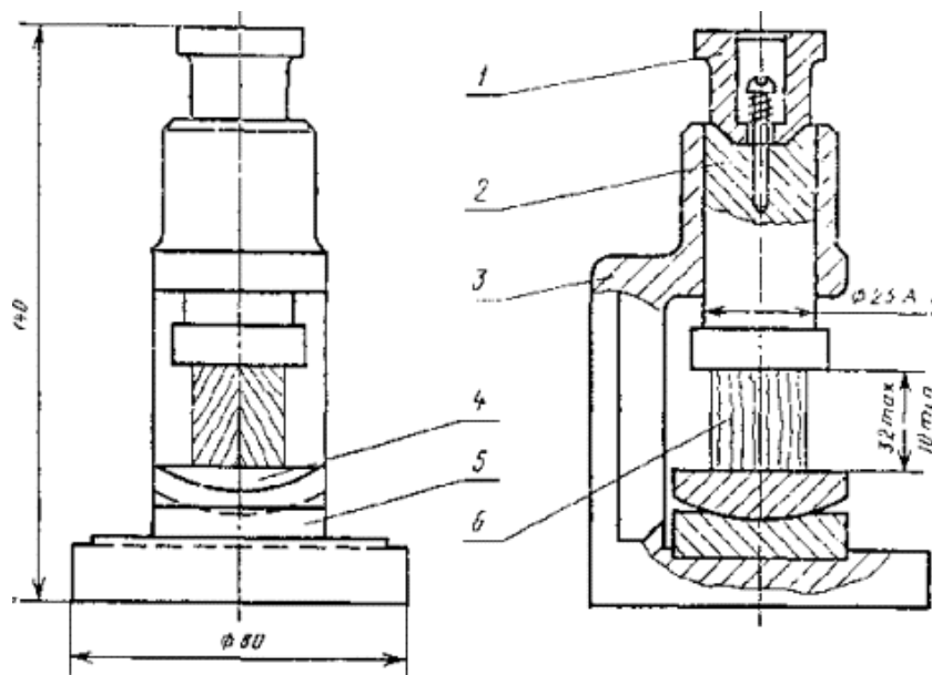
Рис.2. Приспособление к машине для испытания образцов древесины на сжатие вдоль волокон: 1 - колпачок; 2 – пуансон; 3 – корпус; 4 – шаровая опора; 5 – плита; 6 – образец
