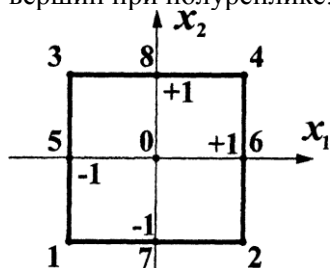
Рис. 7.1. Представление опытов плана В2 на факторной плоскости
