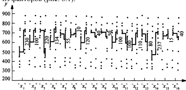
Рис. 8.1. Диаграмма рассеяния
