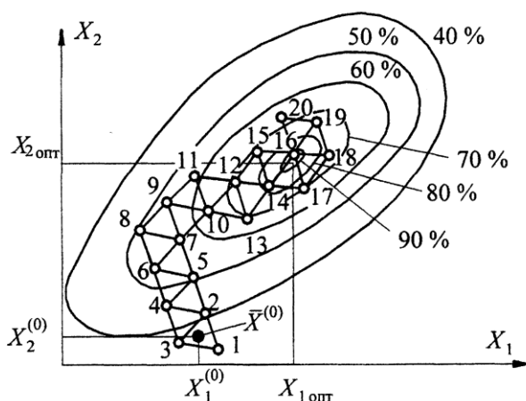
Рис. 9.8. Отыскание максимума функции двух переменных X_1 и X_2
