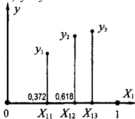
Рис. 9.3. К обоснованию метода золотого сечения
