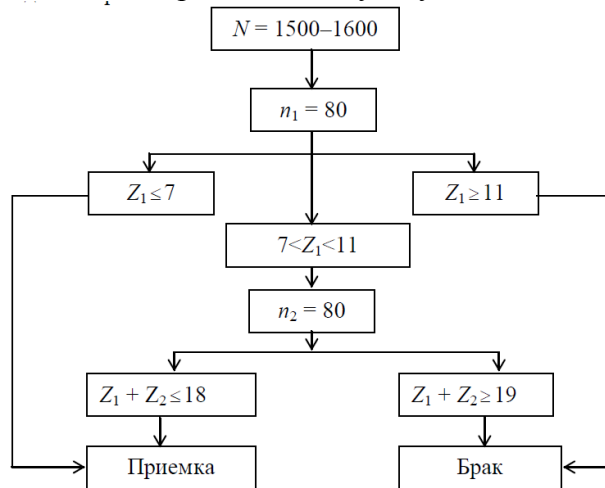
Рис. 3. Последовательность двухступенчатого контроля
