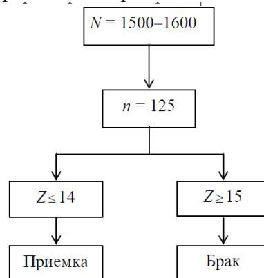
Рис. 2. Последовательность одноступенчатого контроля
