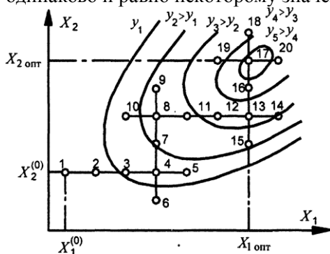
Рис. 9.4. Геометрическая иллюстрация метода покоординатного поиска
