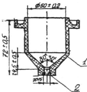
Рис. 2.2. Вискозиметр ВЗ-4.
