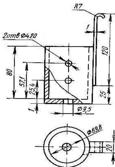
Рис. 3.1 Стандартная кружка ВМС для определения вязкости поливинилацетатной дисперсии
