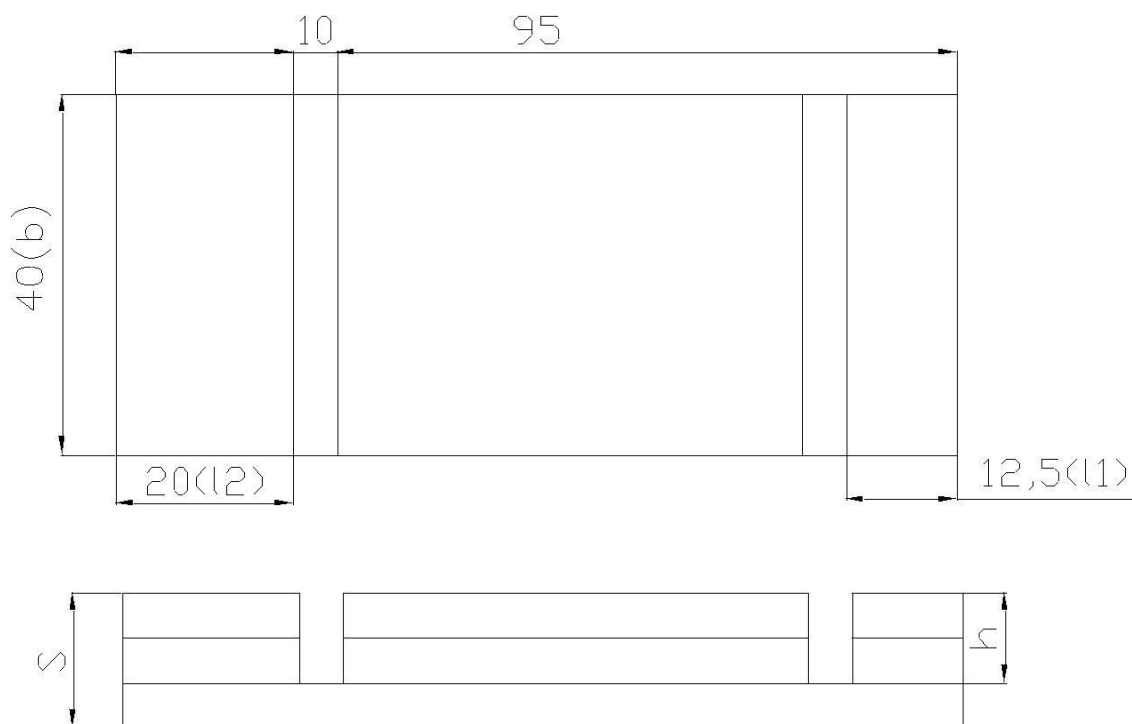
Рис. 2.4. Схема образца фанеры для испытания на скалывание по клеевому слою
