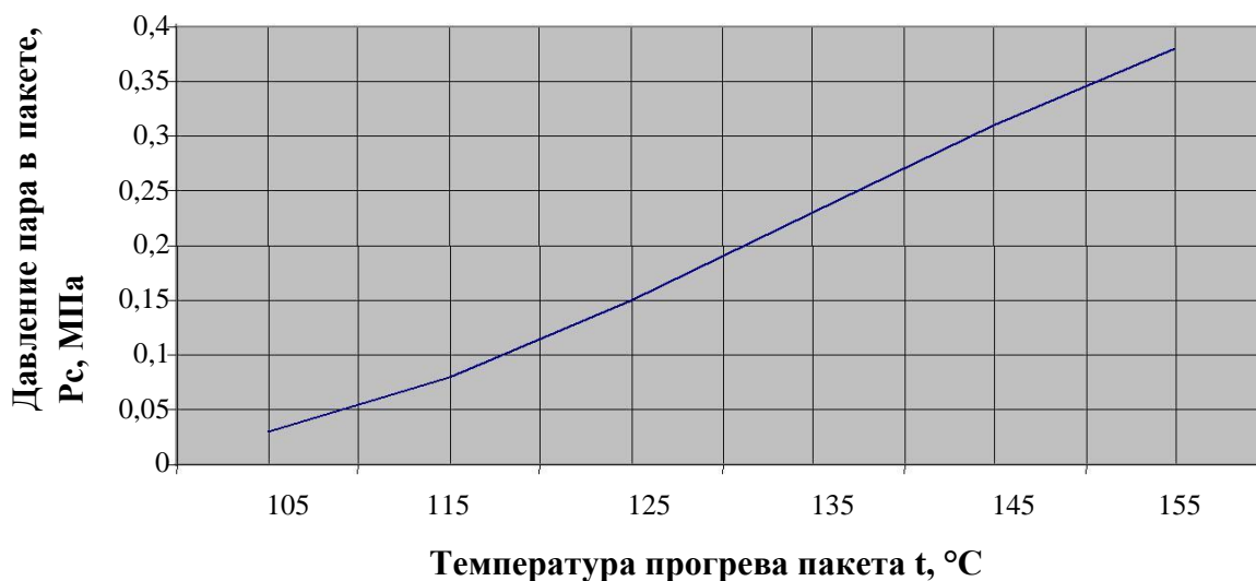
Рис. 2.3 Давление насыщенного пара в пакете при его нагреве
