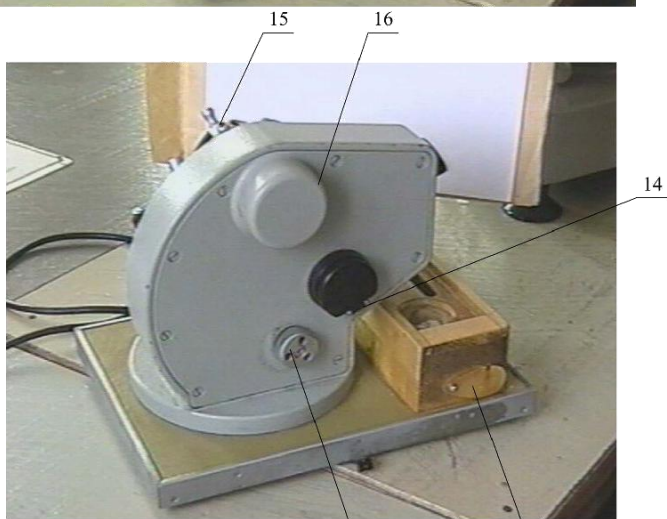
Рис.2.4. Внешний вид рефрактометра Аббе типа ИРФ-22
