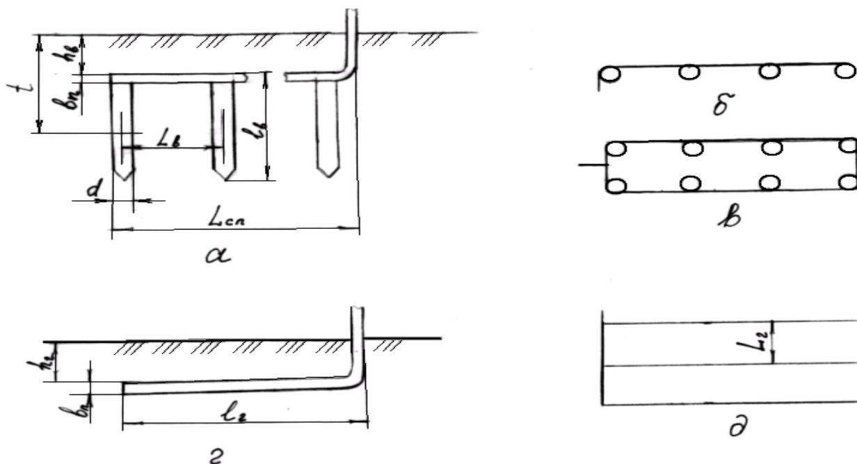
Рис. 1. Заземлительные устройства
