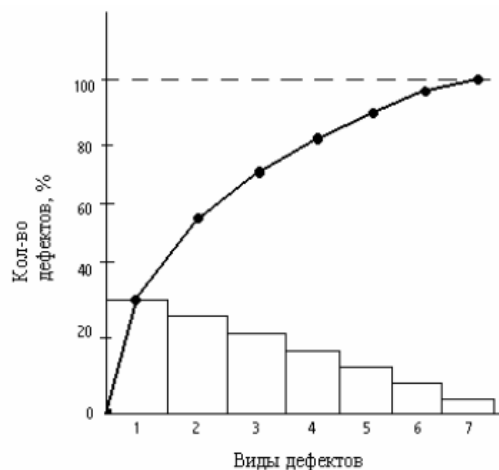
Рис.1.3 Диаграмма Парето для анализа брака
