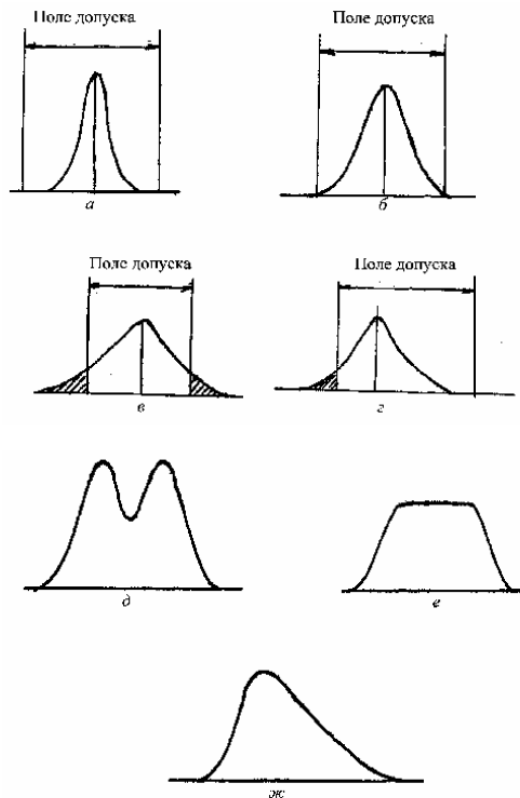
Рис.1.2 Кривые распределения
