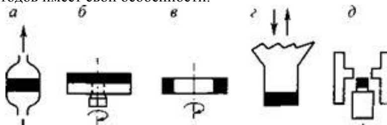
Рис. 11. Варианты определения адгезионной прочности покрытий методом одновременного отрыва:
