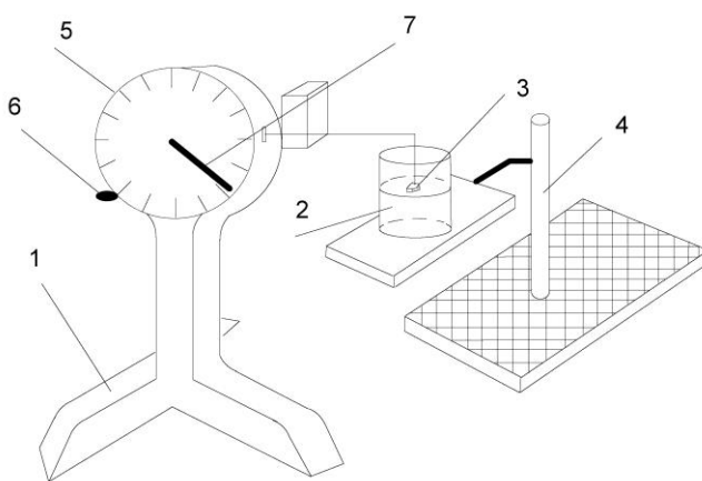
Рис. 1.1. Установка для определения поверхностного натяжения
