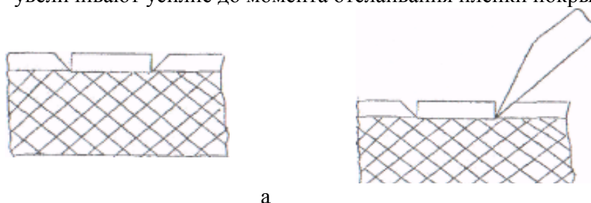
Рис. 13. Схема надрезов лакокрасочного покрытия и определение усилия
