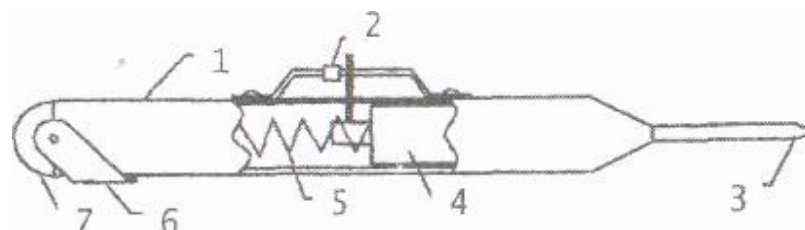
Рис. 12. Общий вид прибора АР-1М:
