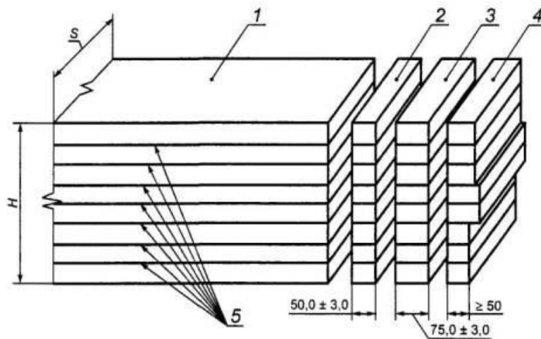
Рис. 1 Принципиальная схема выпиливания образцов для испытаний H - высота клееного элемента; S – ширина клееного элемента; 1 - многослойный элемент ДКК; 2 -заготовка для выпиливания образцов для предварительных испытаний по ГОСТ25884; 3 - образец для испытаний на расслаивание; 4 - торцевой срез; 5 – клеевые швы
