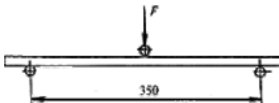
Рис. 5. Схема испытания образцов на прочность при изгибе при постоянном пролете
