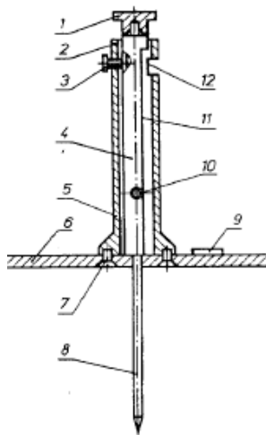
Рис.4 Толщиномер игольчатый
