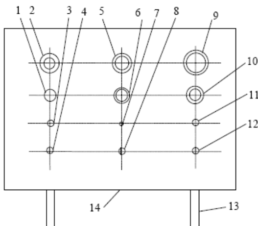
Рис. 8. Шкала гибкости: 1- 12 – стержни; 13 – трубка; 14 – панель
