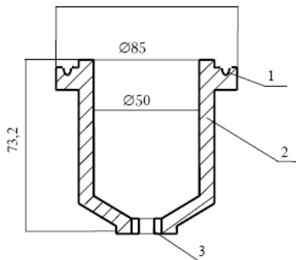
Рис.6. Вискозиметр ВЗ-4:
