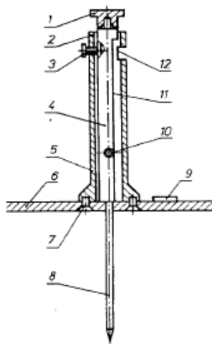
Рис.4 Толщиномер игольчатый
