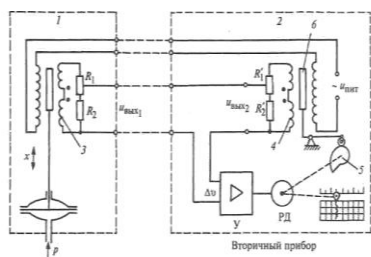
Рис1 Схема дифференциально-трансформаторной измерительной системы:
