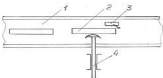
Рисунок 1- Сбрасыватель продольного транспортера
