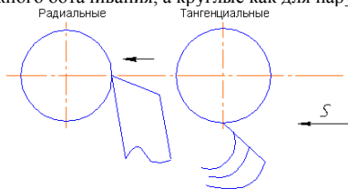
Рис. 4. Схемы подач фасонных резцов
