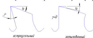
Рис. 17. Форма зубьев фрезы.
