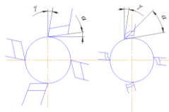
Рис. 24. Схема работы резьбонарезной гребенки
