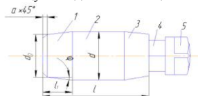
Рис. 13. Общий вид развертки.
