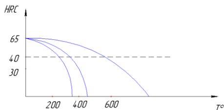
Рис. 1. Зависимость твердости от температуры
